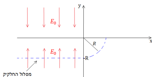
מסלול החלקיק
